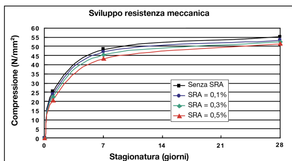
FIG. 3 - Τιμές κονιάματος με βάση το τσιμέντο τύπου CEM I 52,5 R, τυποποιημένη άμμο και νερό, σύμφωνα με τη σύνθεση του προτύπου EN 196-1
