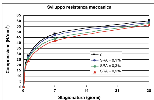
FIG. 4 - Τιμές κονιάματος με βάση το τσιμέντο τύπου CEM I 52,5 R, τυποποιημένη άμμο και νερό, σύμφωνα με τη σύνθεση του προτύπου EN 196-1 με προσθήκη 7% Expancrete
