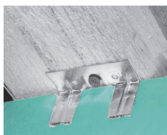
Διαδικασία εφαρμογής θερμομόνωσης FIBRANxps MAESTRO με μη εμφανή στηρίγματα
